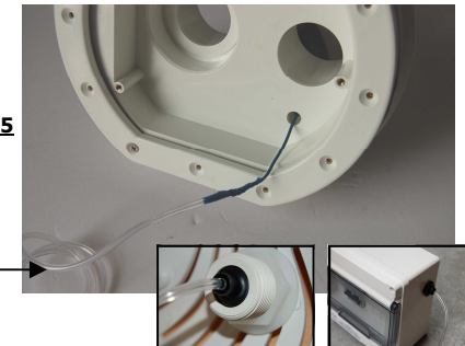
Tube de commande Pneumatique/ Pneumatic control pipe/Tubo de control neumático
